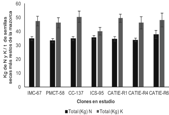
Figura 1. Extracción total de nitrógeno y potasio por tonelada de semillas secas y los restos de la mazorca en siete clones de cacao en dos localidades de Costa Rica. Octubre, 2014.
