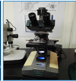
Figura 4. Estereoscopio (A) Cámara de conteo de larvas y huevos (B) Microscopio de luz para lectura C. INTA. 2020.
