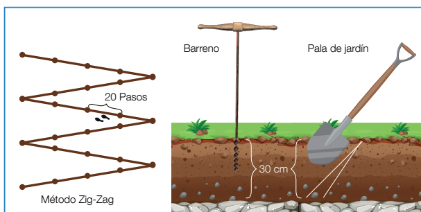
Figura 1. Sistema de muestreo en campo (A y B). INTA, 2015. CIP, 1986.
