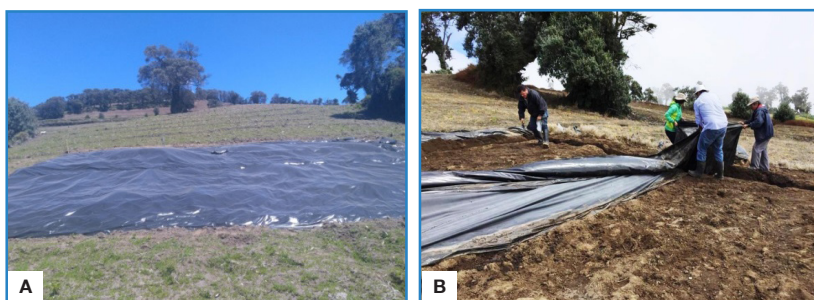
Figura 6. Instalación plástico (A), separación del polietilenotricapa (B). Cartago. 2019.
