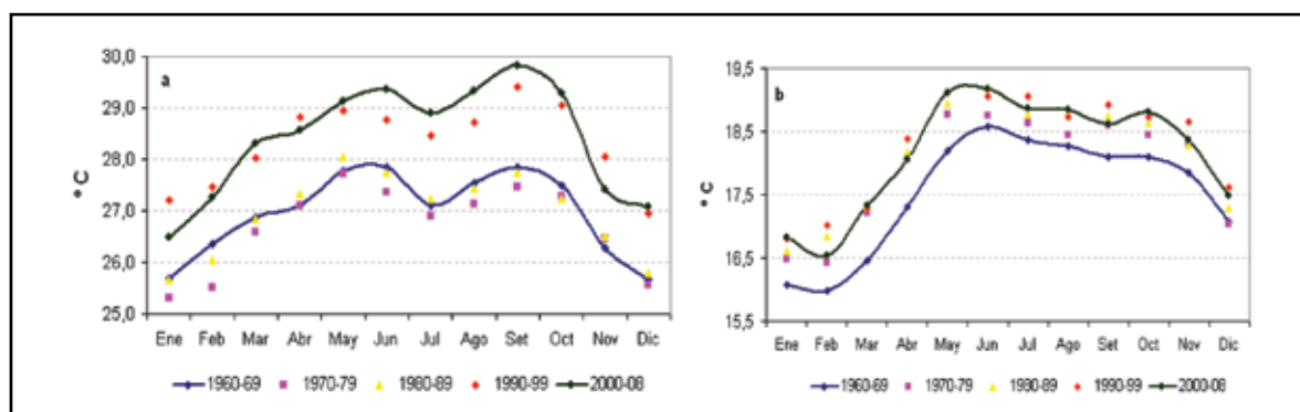
Figura 3 (a) y 3 (b). Temperatura a) máxima y b) mínima, diaria mensual promedio por década. Turrialba, Costa Rica. Periodo 1960 – 2008. 2008.
