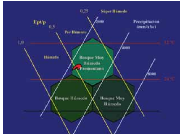
Figura 4. Desplazamiento de Turrialba en la zona de vida de Bosque Muy Húmedo Pre montano Tropical. Turrialba, Costa Rica. 2008.
