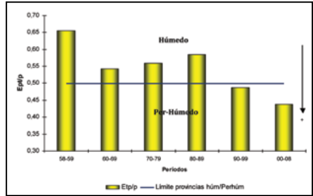
Figura 3. Evaporación potencial en diferentes períodos y límites de provincias de humedad, de acuerdo con la clasificación de Zonas de Vida de Holdridge (1978). Turrialba: 1958-2008. 2008.
