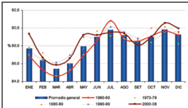
Figura 7. Humedad relativa promedio anual por período. Turrialba 1960 – 2008. Turrialba, Costa Rica. 2008.
