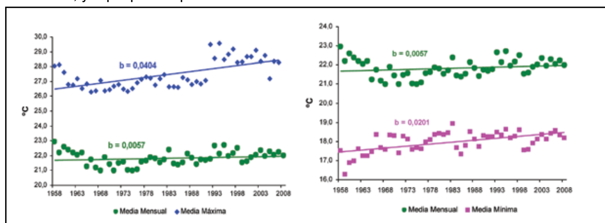
Figura 1. Temperatura media, media máxima y media mínima mensual por año. Turrialba, Costa Rica. Periodo 1958-2008. 2008.
