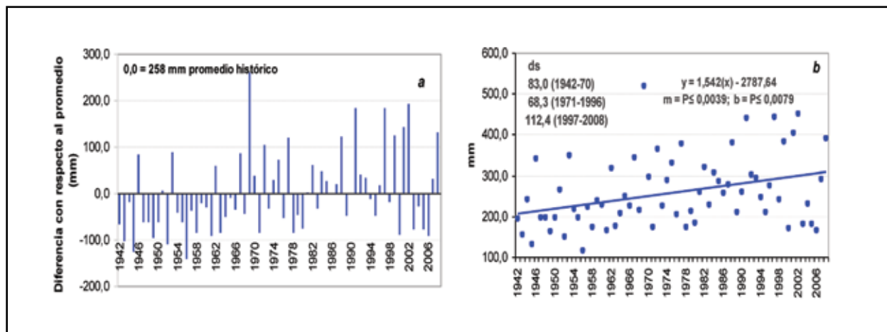
Figura 5. Variación de la precipitación del mes de agosto, a) con relación al promedio histórico del mes; b) en el periodo de 67 años. Turrialba, Costa Rica. 2008.
