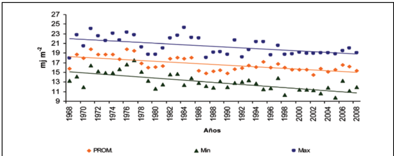
Figura 7. Radiación solar promedio, máxima y mínima promedio anual. Turrialba, Costa Rica. Periodo 1968 – 2008. 2008
