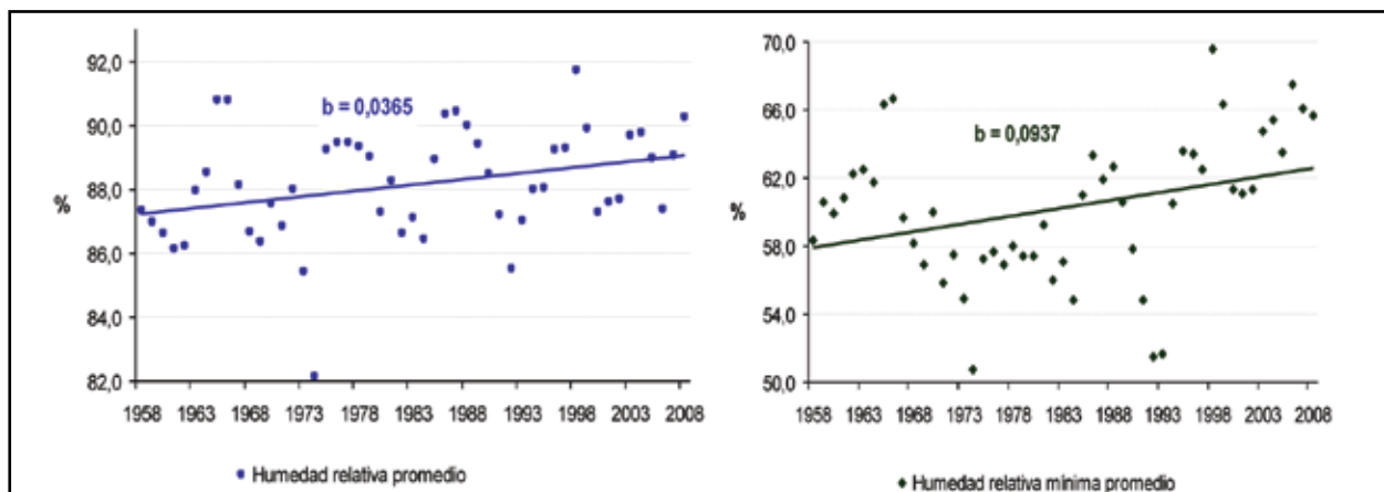
Figura 6. Humedad relativa promedio y mínima promedio anual. Turrialba, Costa Rica. Periodo 1958 – 2008. 2008.
