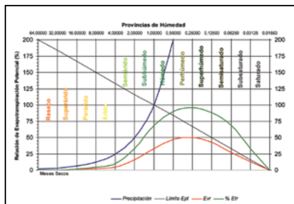
Figura 1. Diagrama de movimiento de agua en asociaciones climáticas (Holdridge 1963)
