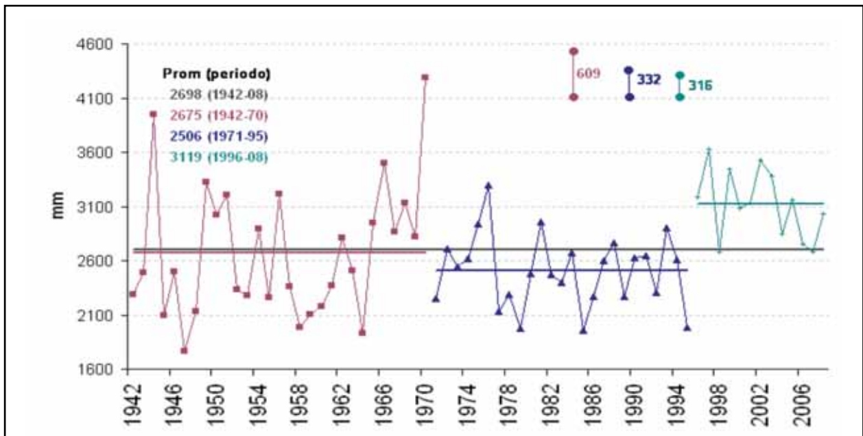
Figura 4. Precipitación promedio en tres periodos, desde 1942 hasta el 2006. Turrialba. Costa Rica. 2008.
