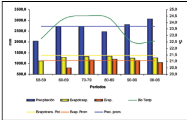
Figura 6. Precipitación, evaporación, bio temperatura y evapotranspiración estimada, de acuerdo con el sistema de clasificación de zonas de vida de Holdridge (1967). Turrialba: 1958 – 2008. Turrialba, Costa Rica. 2008.
