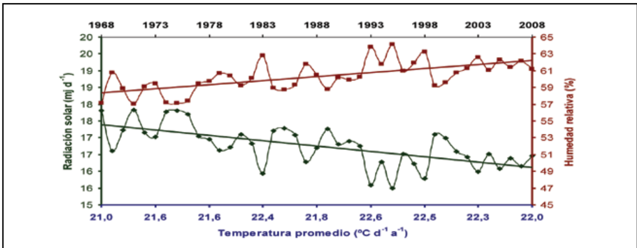
Figura 8. Variación de la radiación solar y la humedad relativa con respecto a la temperatura promedio diaria anual. Turrialba, Costa Rica. Periodo 1968 – 2008. 2008.
