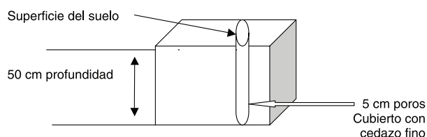
Figura 2. Diseño y colocación en el suelo del dispositivo recolector de agua para determinación de contaminantes. Guanacaste, Costa Rica. 2000.
